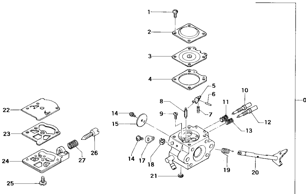
FIG.4 CARBURETOR
